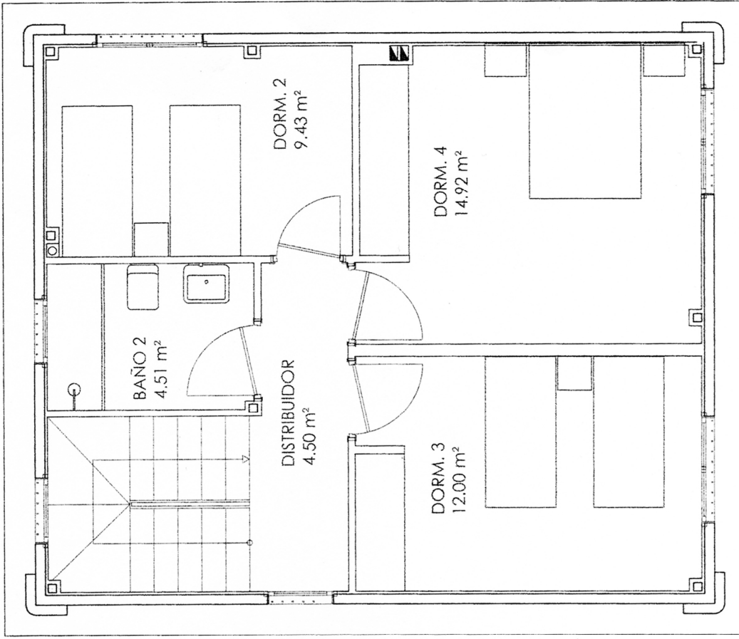
PLANTA PRIMERA
