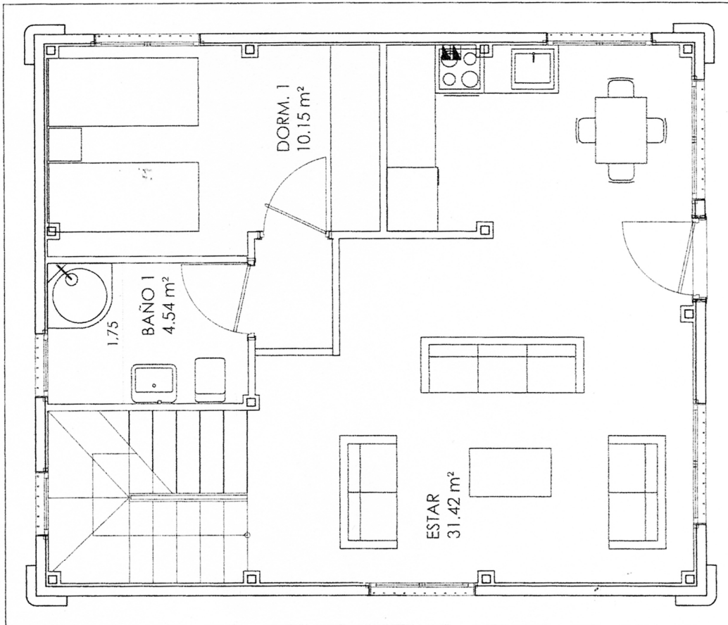
PLANTA BAJA
